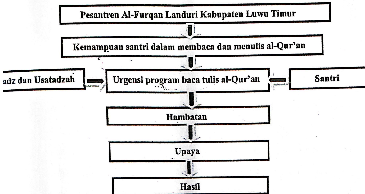
Gambar 2.1 Kerangka Pikir
