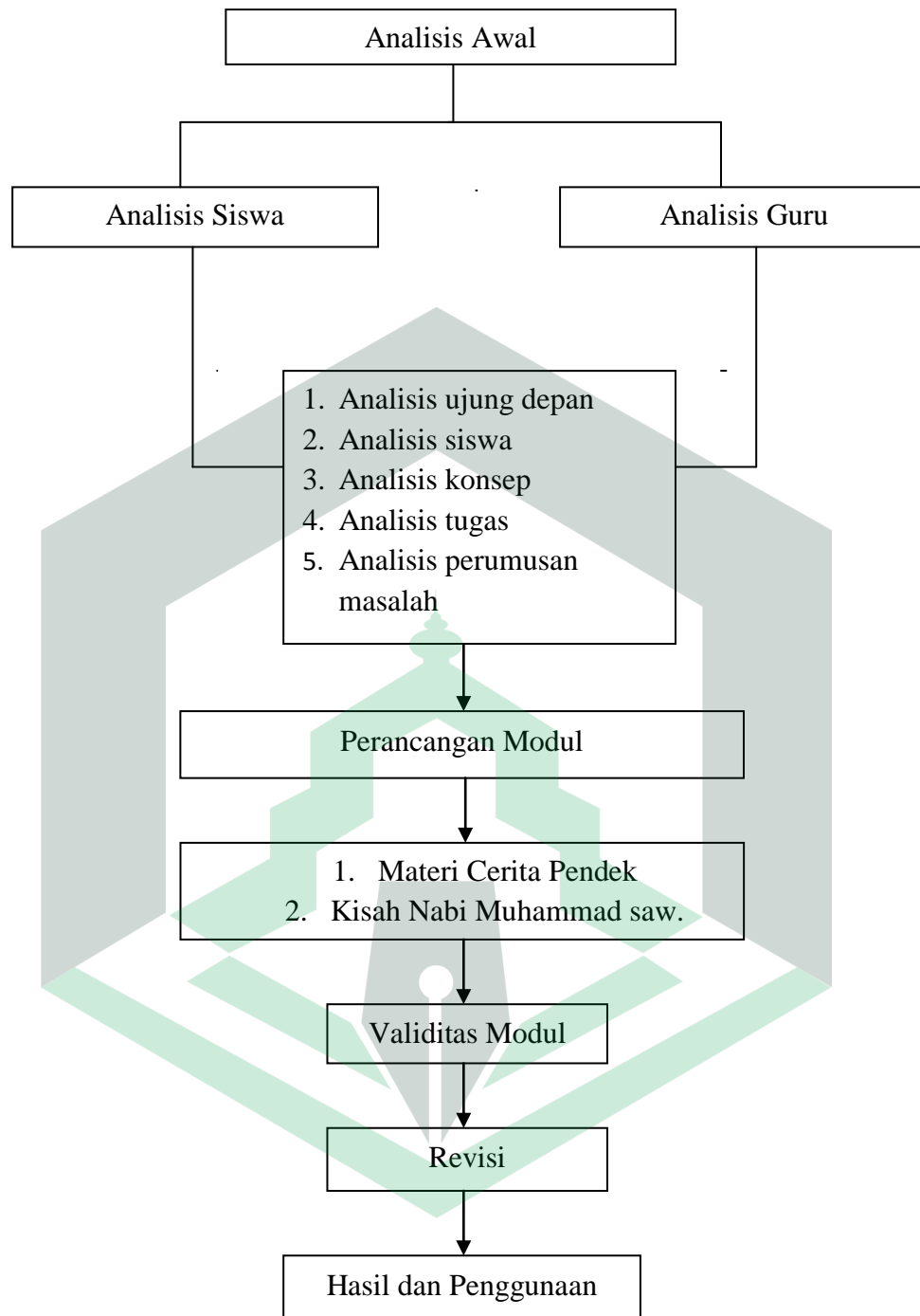
Gambar 2.1: Kerangka Pikir
