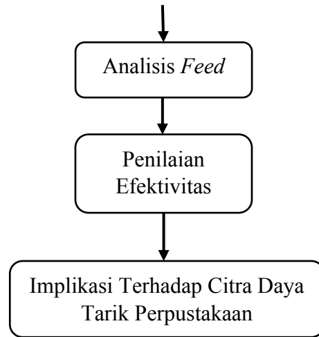
Gambar 2.1 Kerangka Pikir
